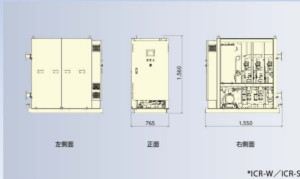
外観図
