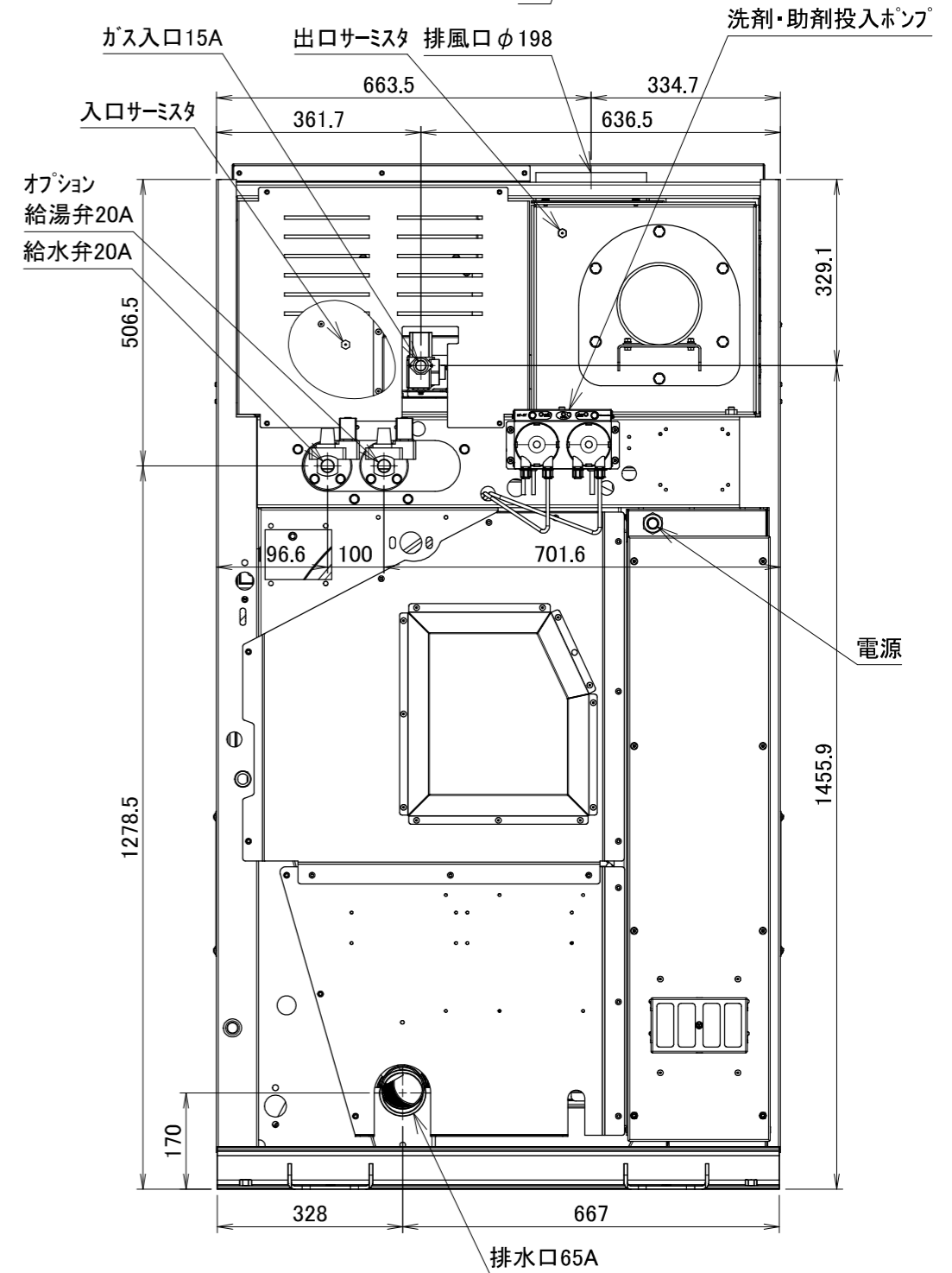
WD272CS外観図
